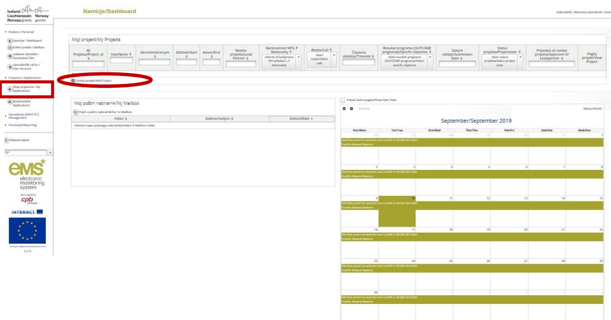
Slika 4: Dodaj projekt
