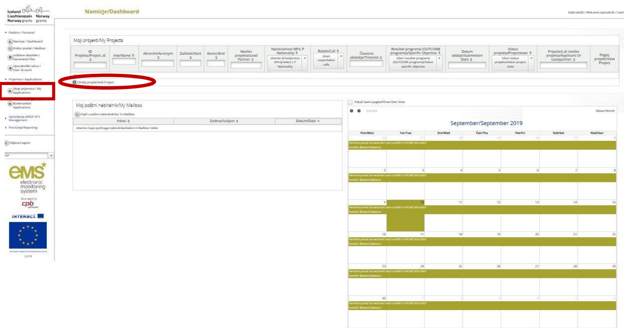
Slika 4: Dodaj projekt
